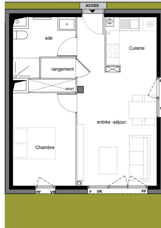
niveau RdC
